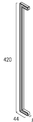
Endkappe 6039
