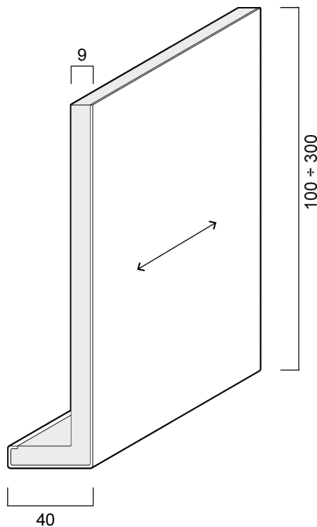
Außenecke 6R36
